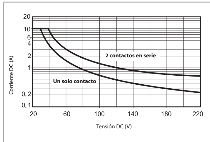
H 40.6 - Máximo poder de corte con cargas en DC1 Tipo 40.62
