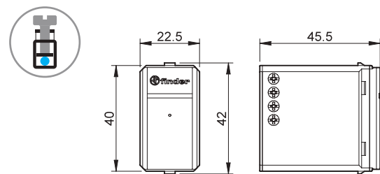
Tipo 15.71 - YESLY Borne de jaula
