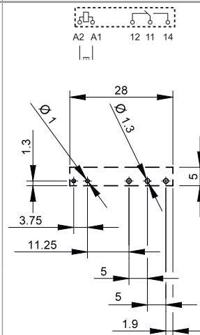
Vista parte inferior
