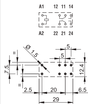
Vista parte inferior Largo de terminal 5.3 mm para CI o zócalos
