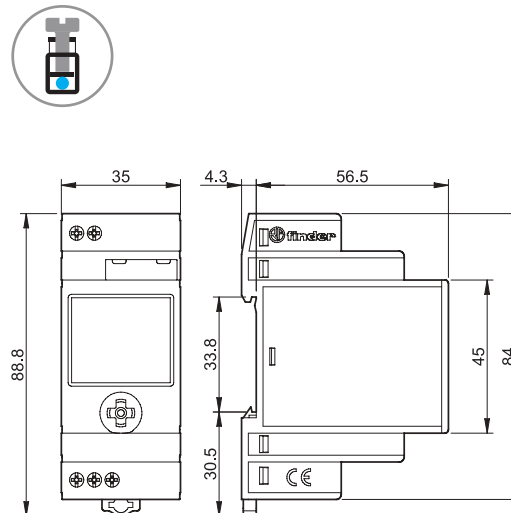
Tipo 12.61 / 12.A1 Borne de jaula
