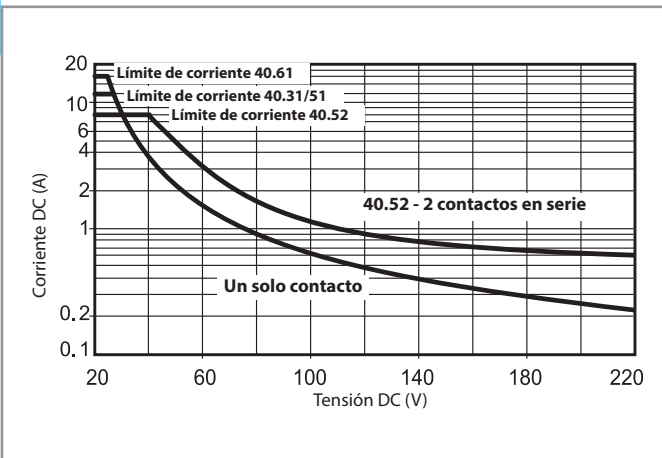
H 40.1 - Máximo poder de corte con cargas en DC1 Tipos 40.31/51/52/61
