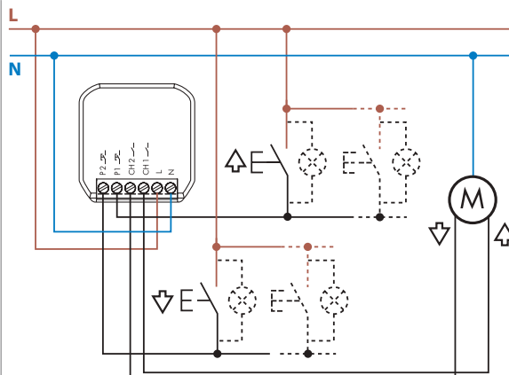
Tipo 13.S2 Conexión a 4 hilos
