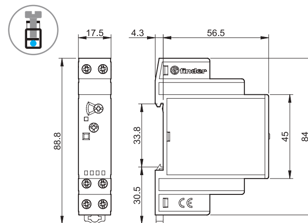
Tipo 15.11 Borne de jaula
