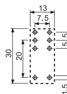
95.15.2 Vista parte inferior
