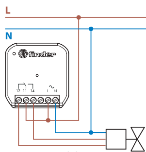
Tipo 13.21.8.230.S000 Electroválvula de 2, 3 y 4 hilos o conexión directa
